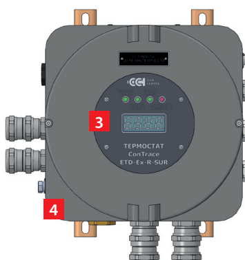
Корпус термостата. Вид спереди
