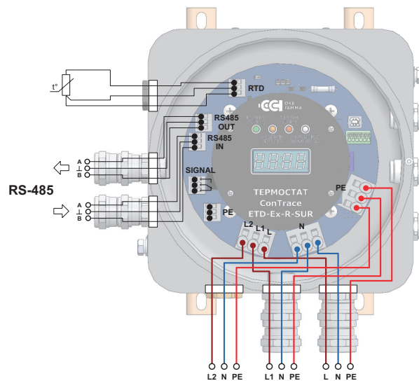
Схема проходного подключения термостата в сети RS-485
