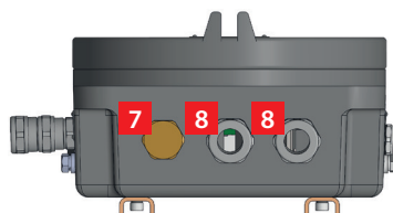
Корпус термостата. Вид снизу
